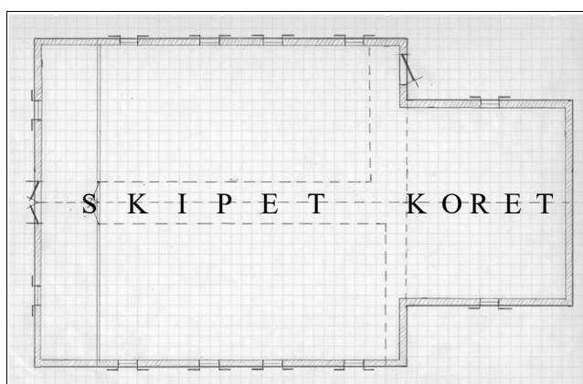
Kirkens grunnplan
