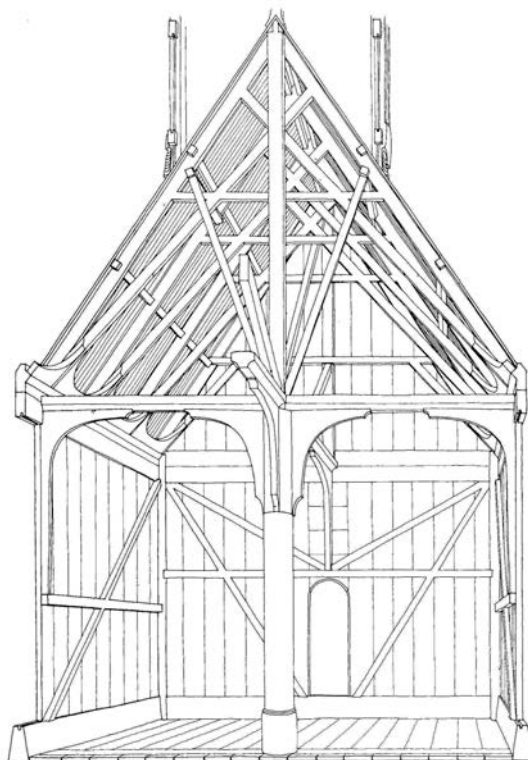
Typisk midtmastkirke
