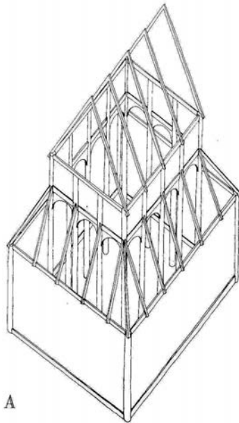
Enkel stavkirkekonstruksjon
